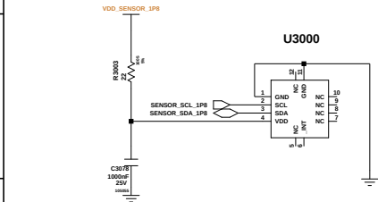
ALS Sensor
