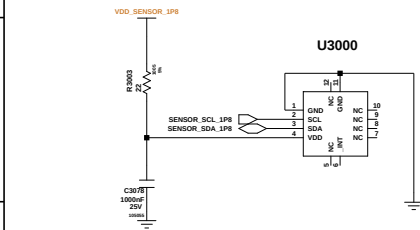
ALS Sensor
